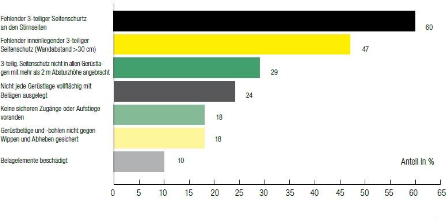
Abb. 21: Ausführungsmängel an Arbeits- und Schutzgerüsten
